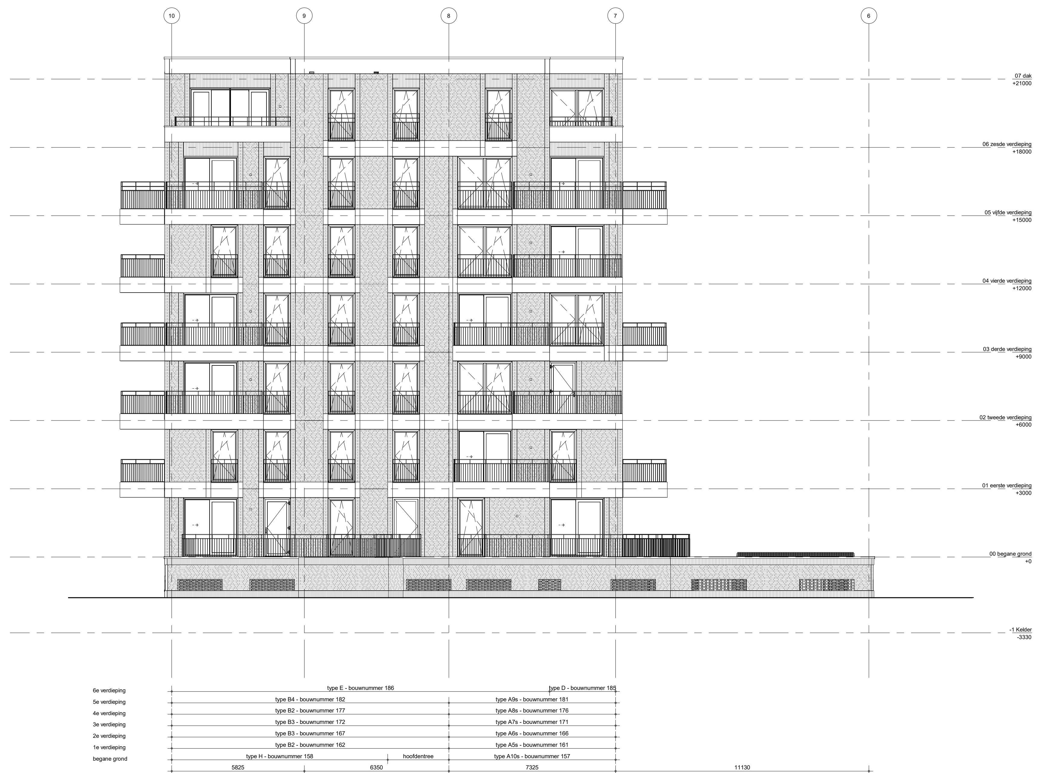
oostgevel
