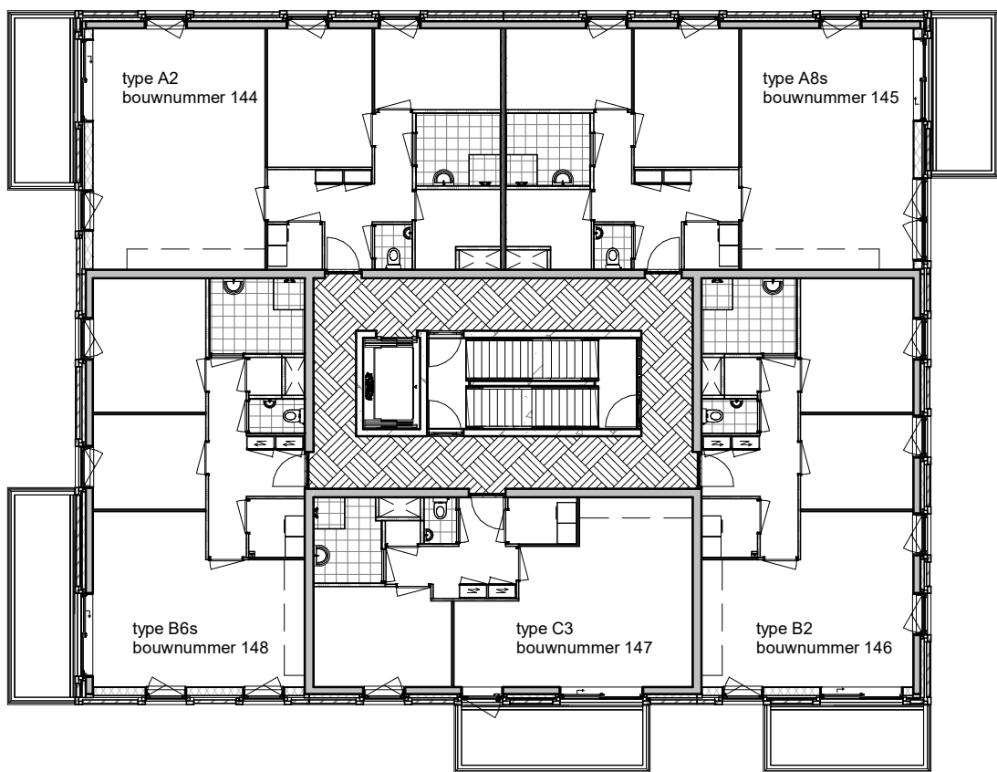
vierde verdieping
