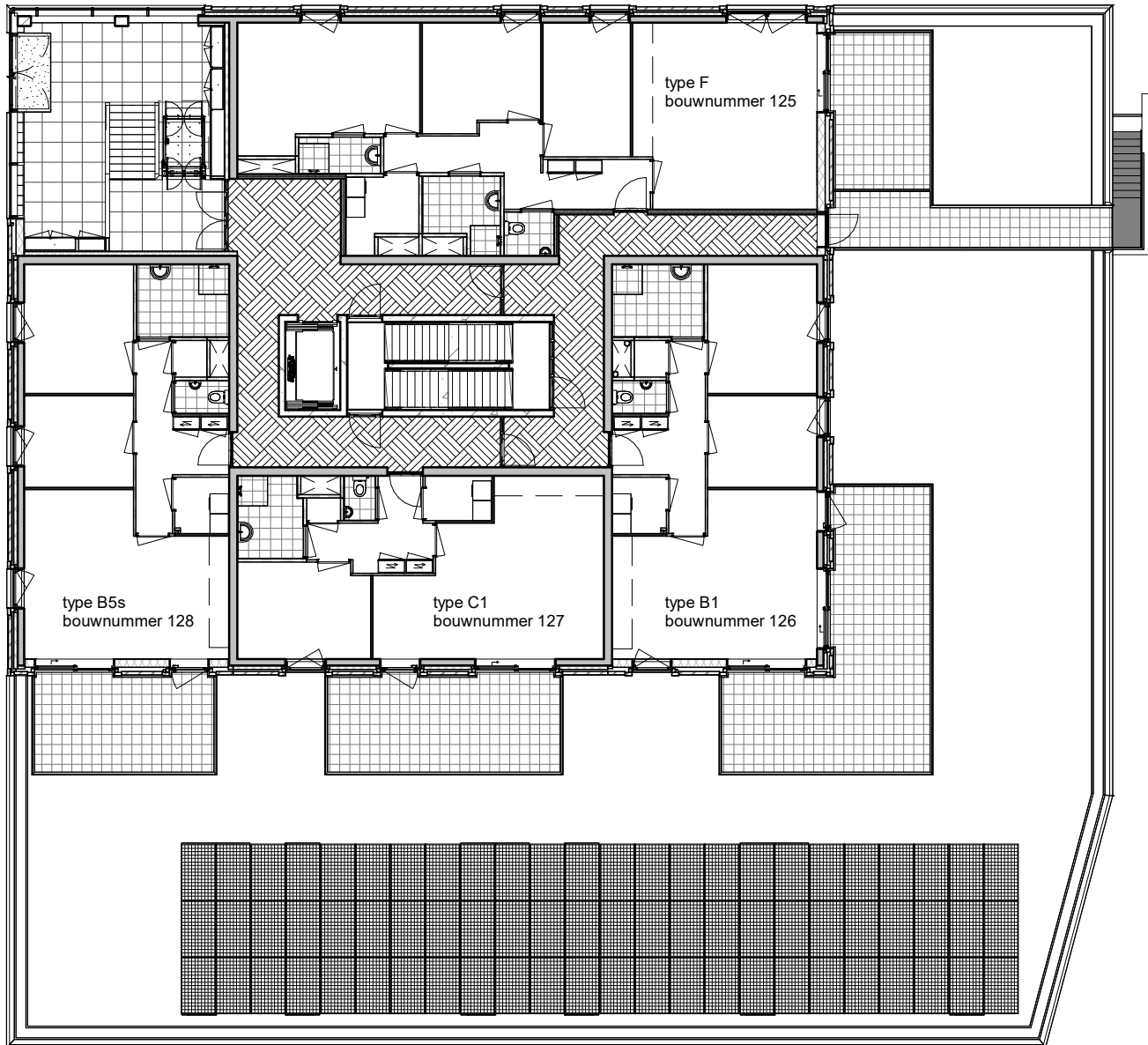
begane grond
