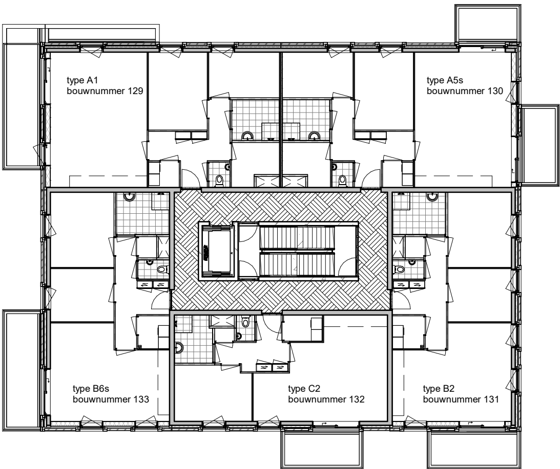
eerste verdieping
