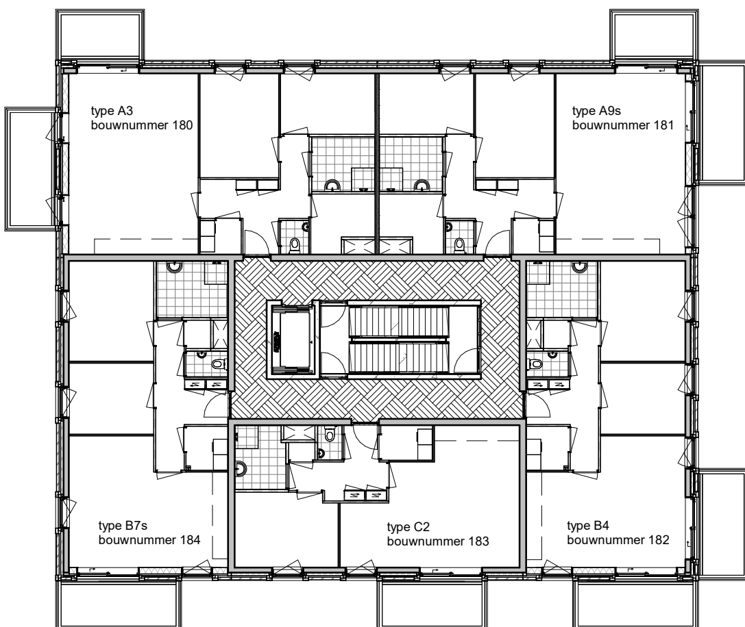
vijfde verdieping
