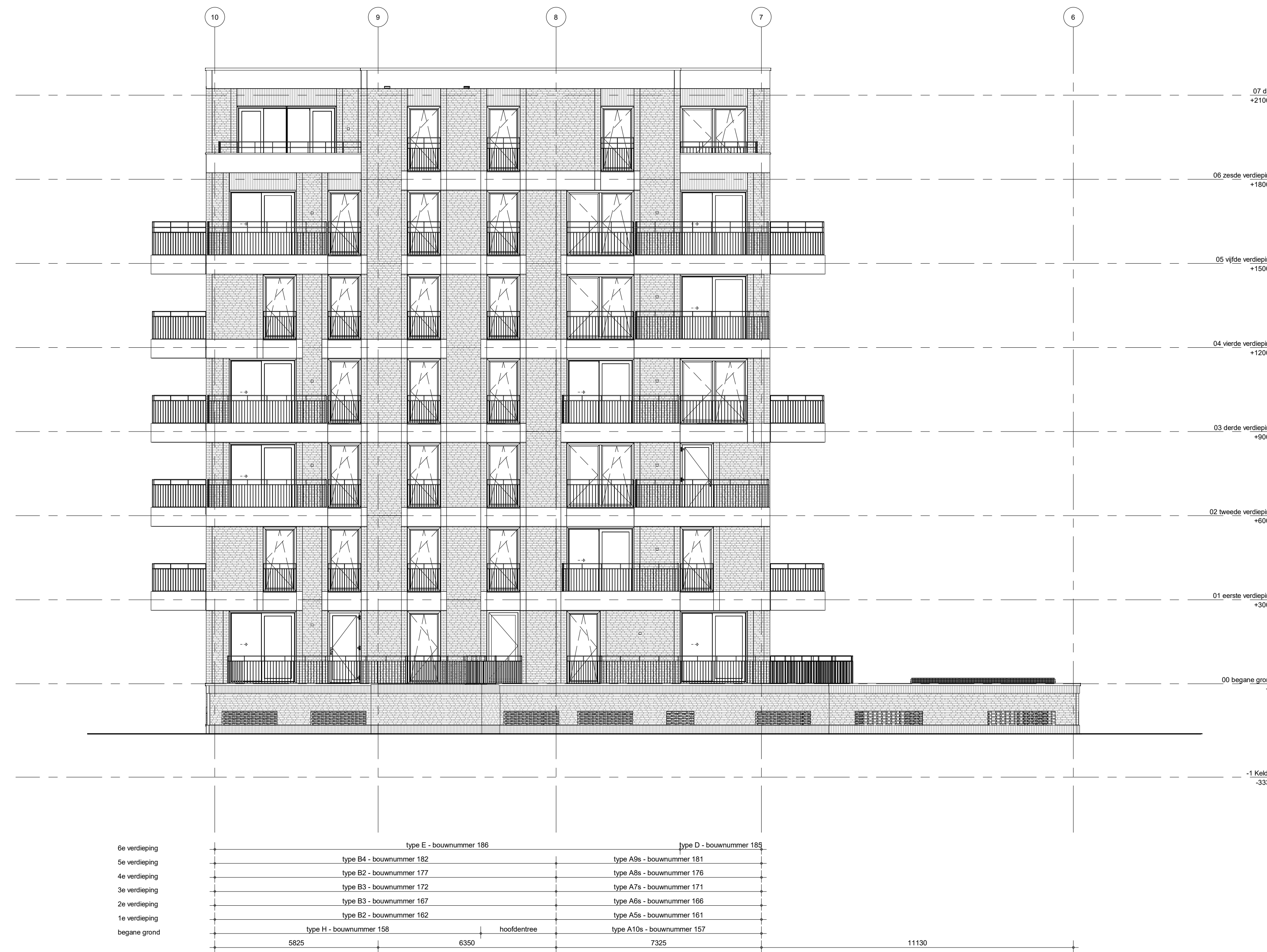
oostgevel
