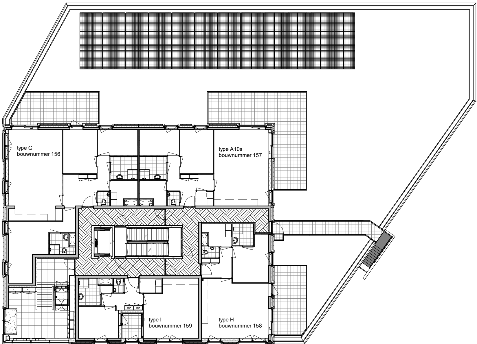
begane grond
