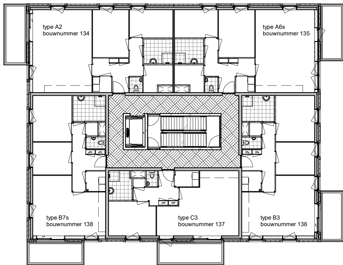
tweede verdieping
