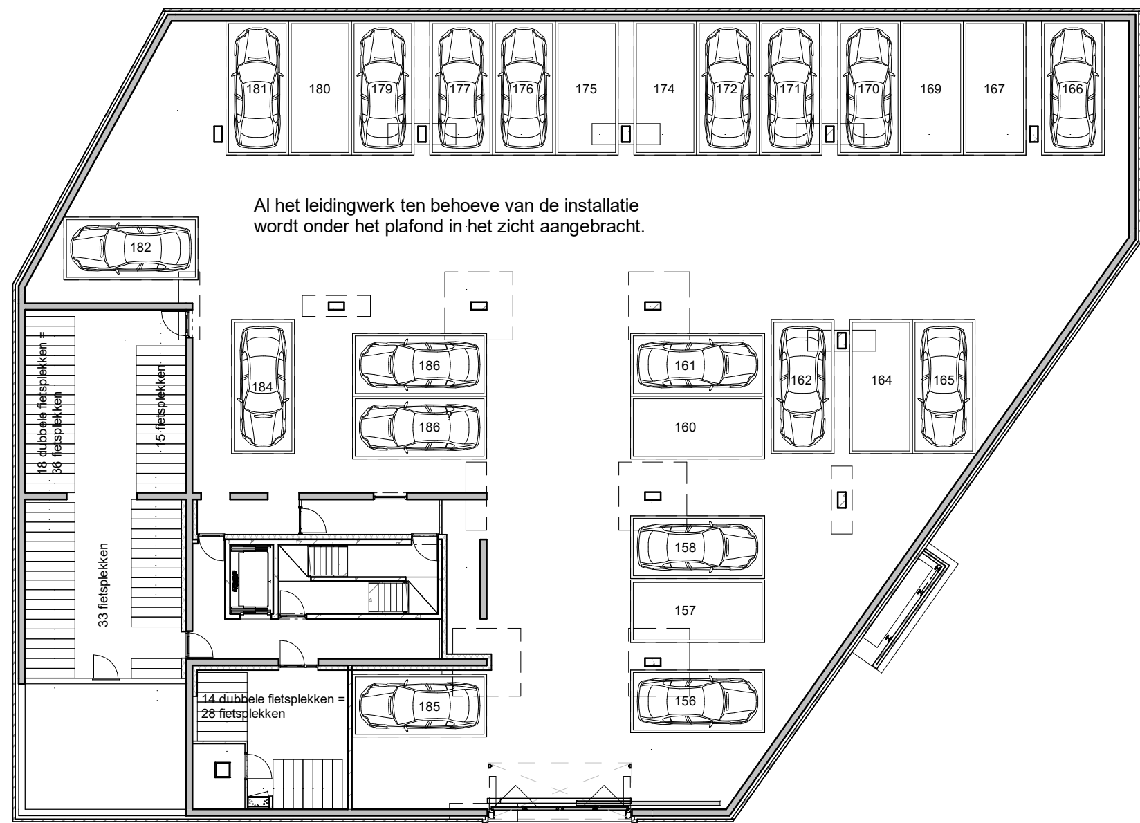
kelder
