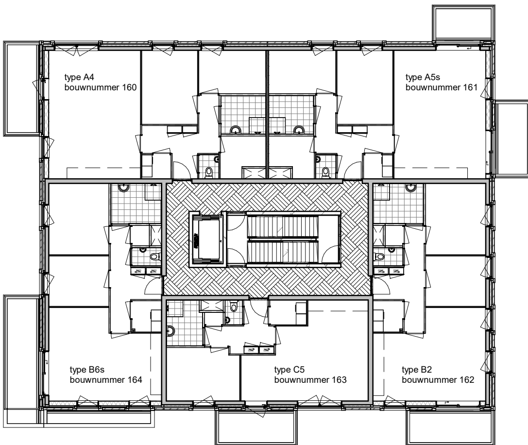
eerste verdieping
