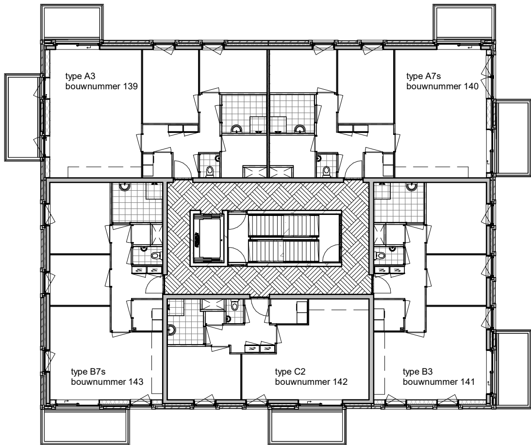
derde verdieping
