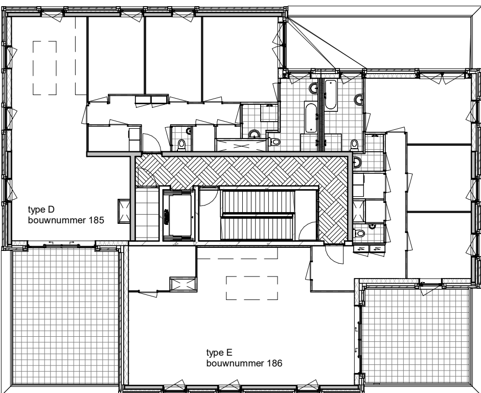
zesde verdieping
