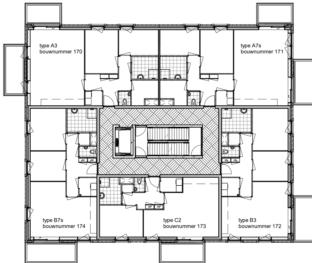
derde verdieping
