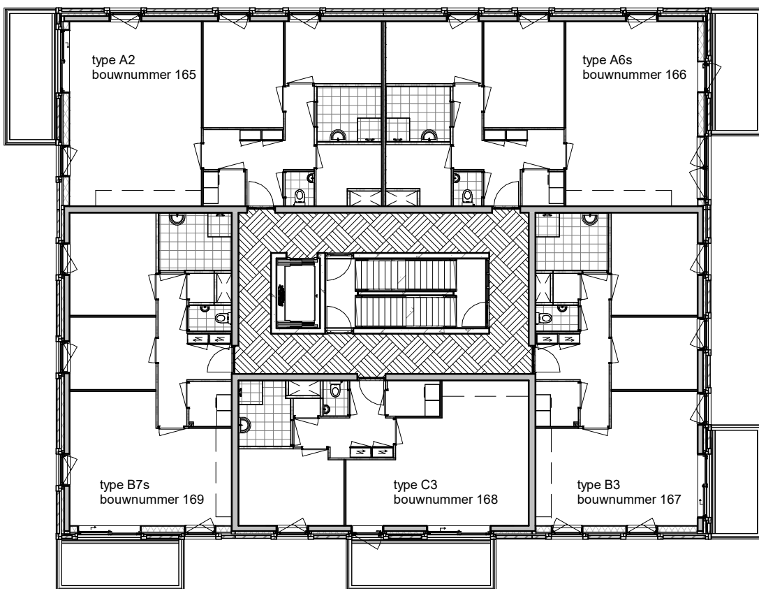
tweede verdieping
