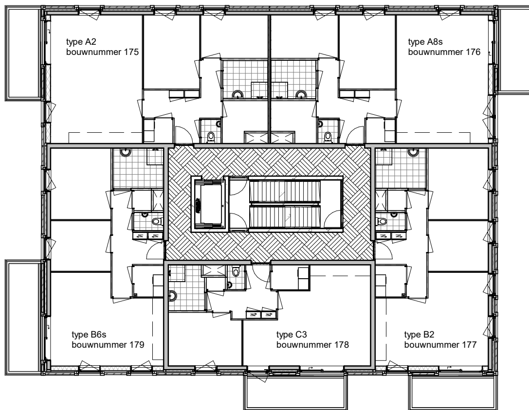
vierde verdieping
